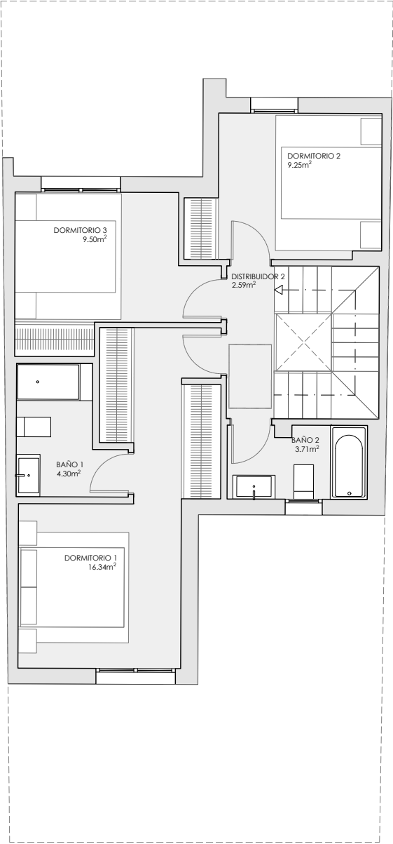
PLANTA PRIMERA
