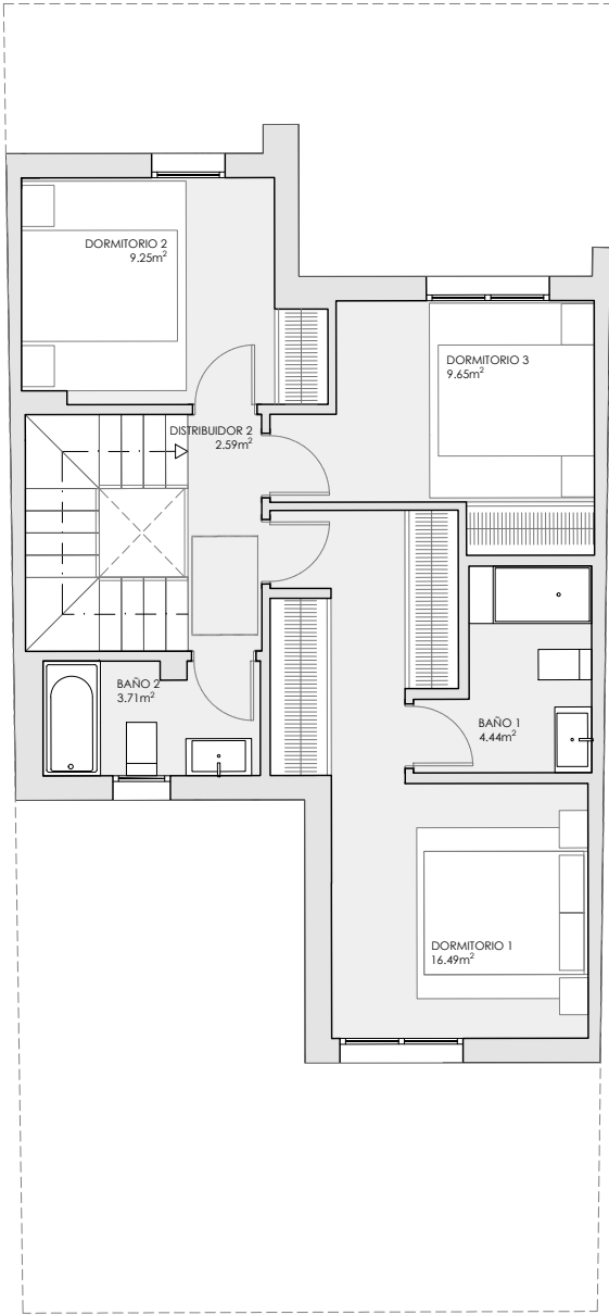
PLANTA PRIMERA
