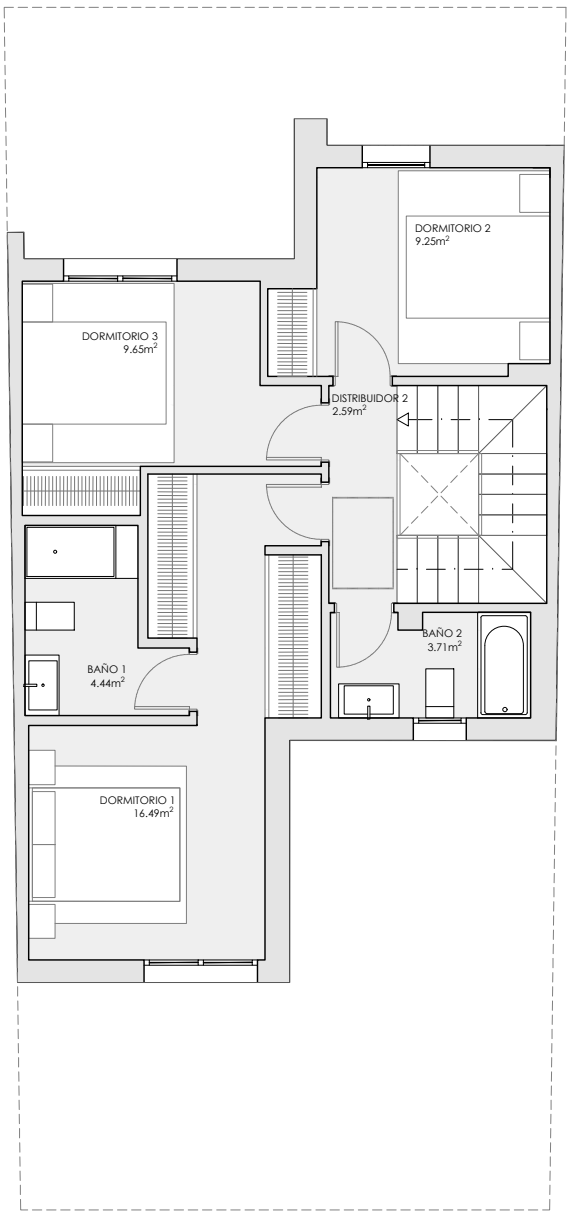
PLANTA PRIMERA
