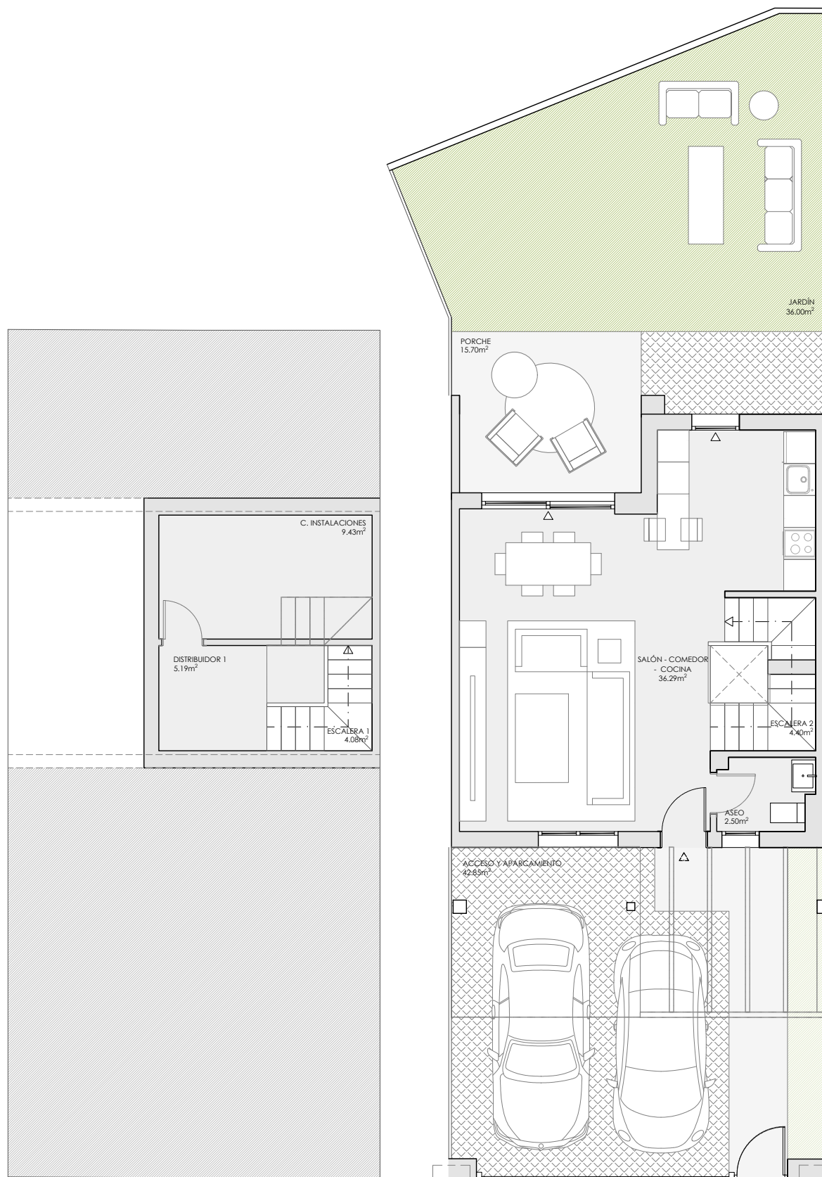
PLANTA SÓTANO
