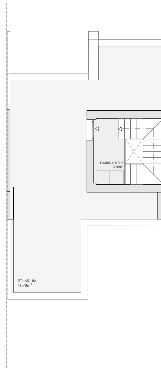
PLANTA CUBIERTA
