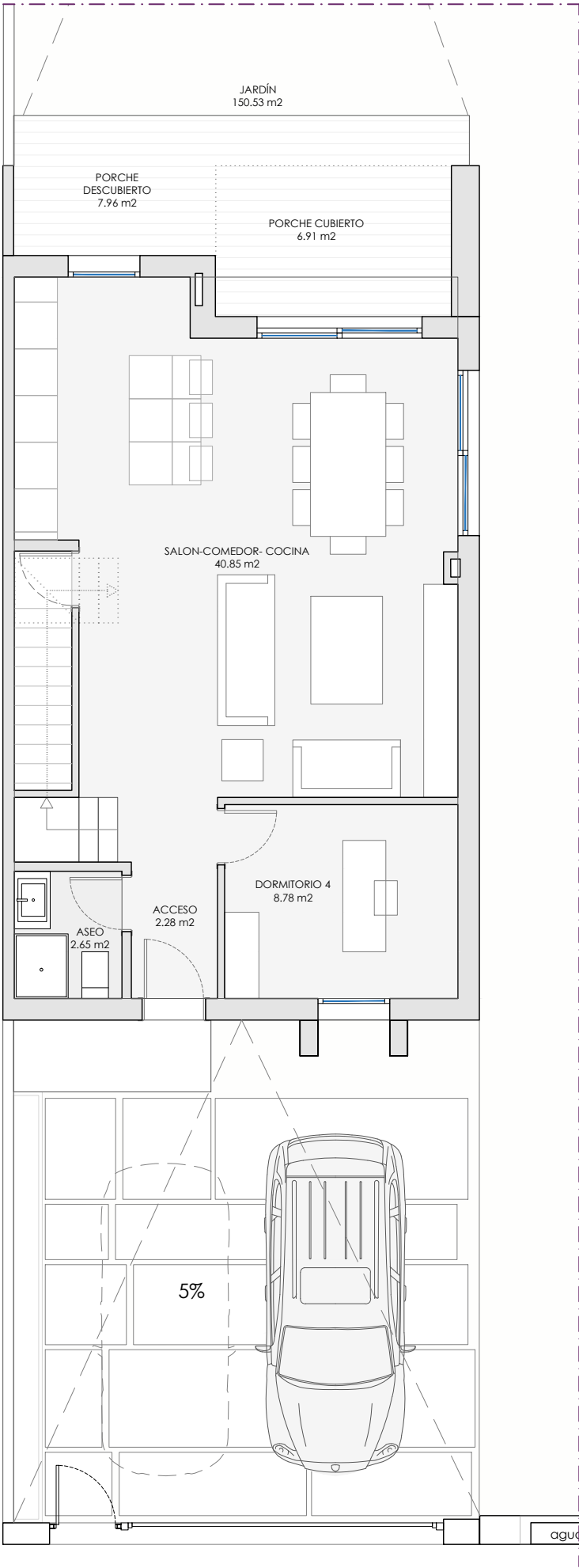
PLANTA BAJA
