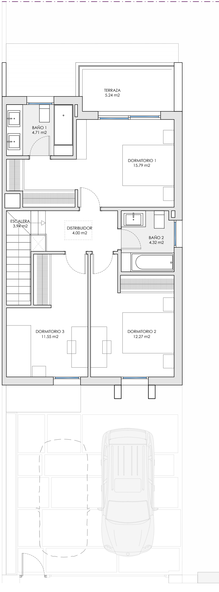
PLANTA PRIMERA
