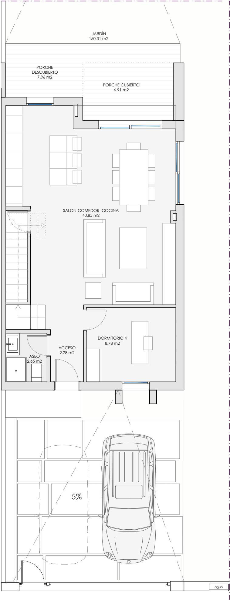
PLANTA BAJA
