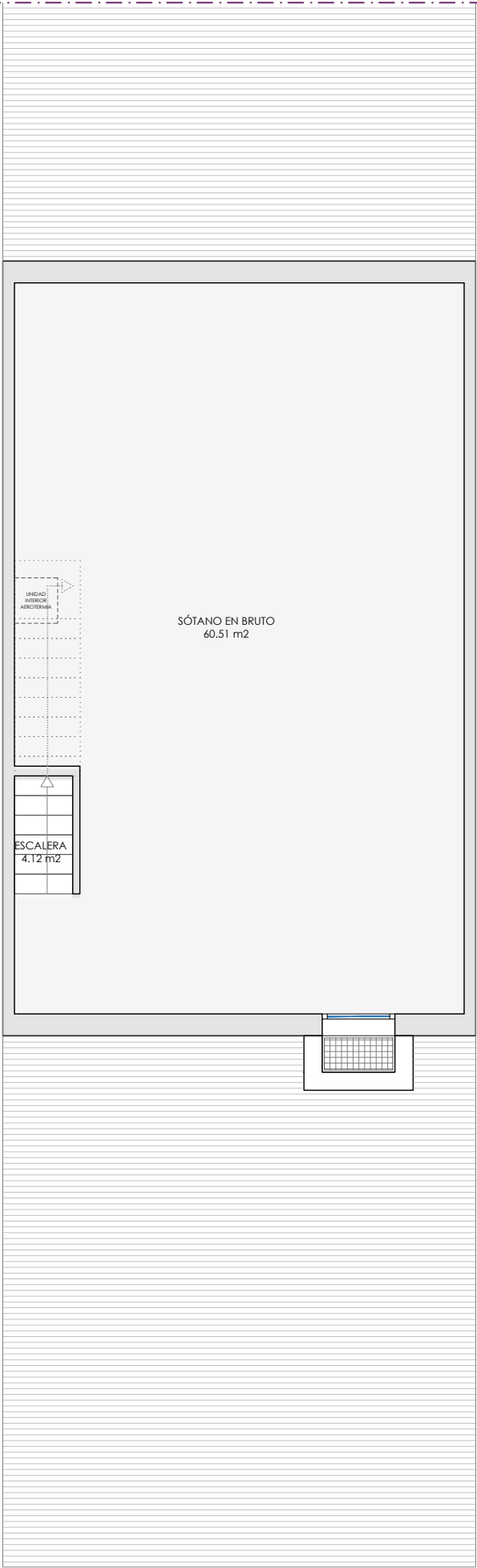
PLANTA SÓTANO
