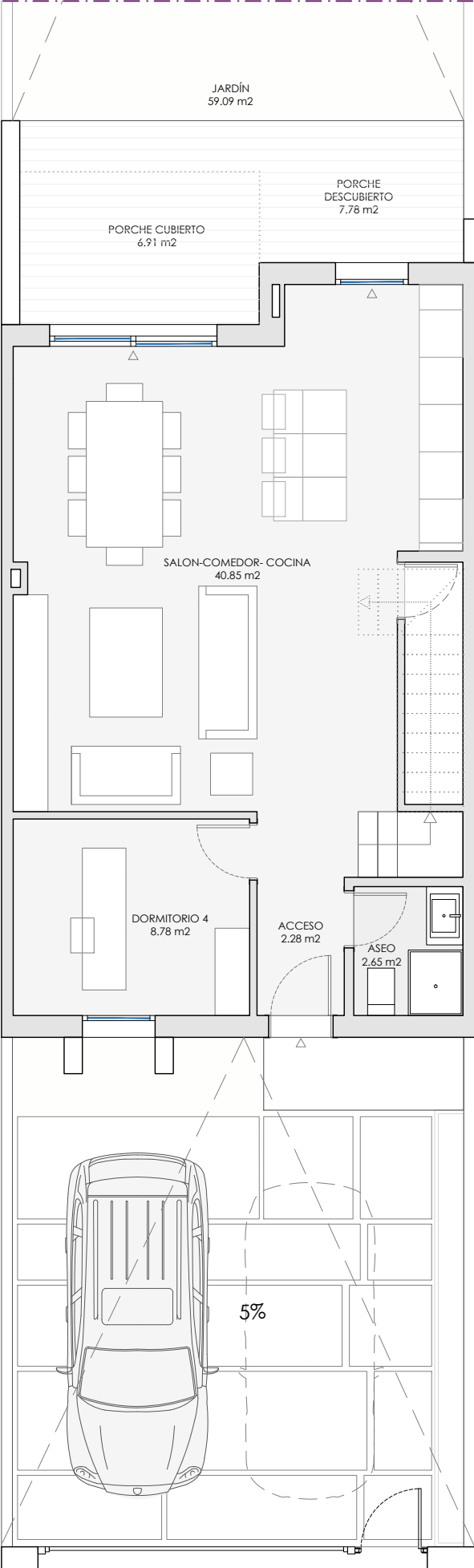
PLANTA BAJA
