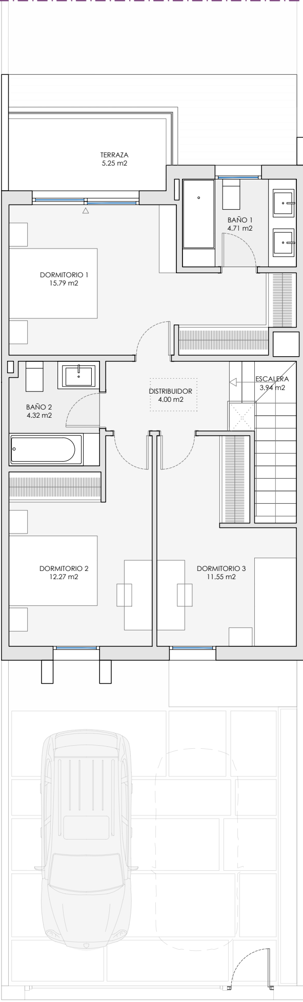
PLANTA PRIMERA
