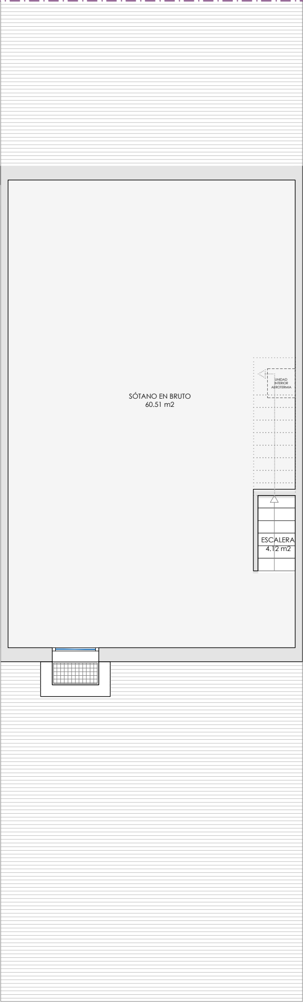
PLANTA SÓTANO
